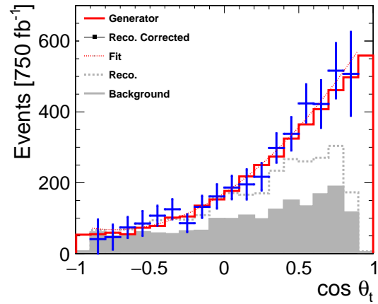
(d) Mid energy, +80% polarization
