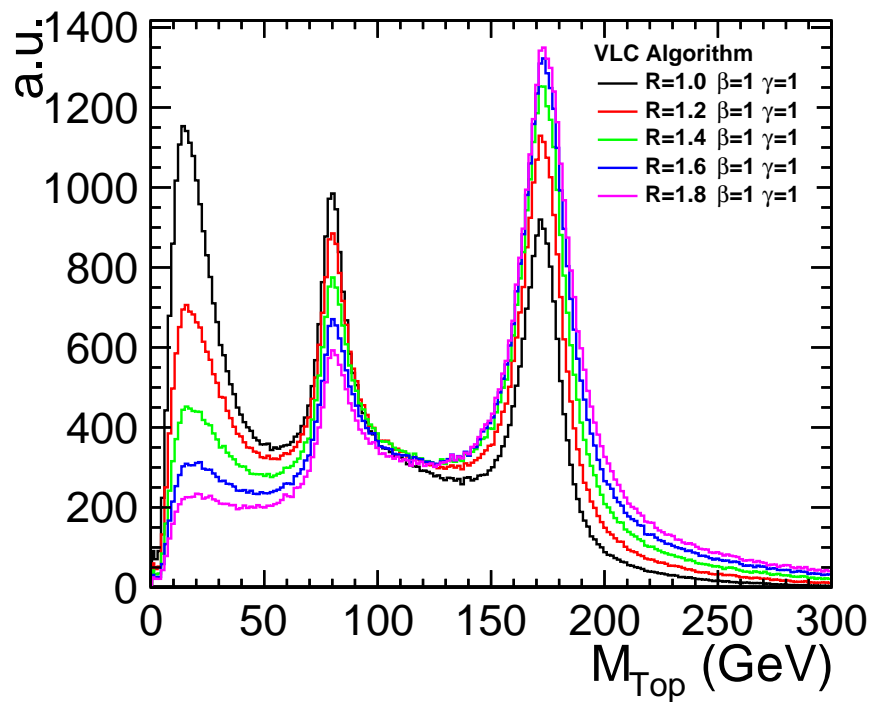
(b) Valencia algorithm
