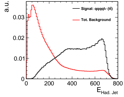
(d) Energy of hadronic fat jet
