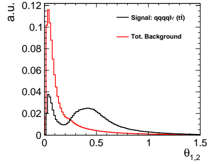
(j) \theta_{1,2}
