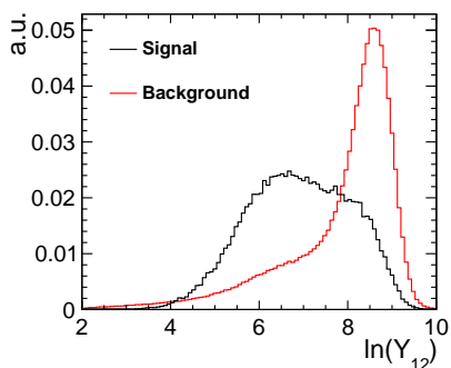
(s) Jet Resolution Parameter Y_{12}
